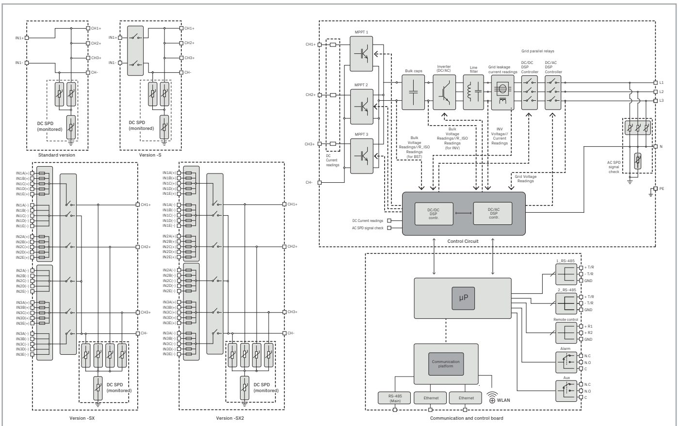
Diagramma a blocchi PVS-50/60-TL
