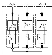
Schema di principio DG M YPV SCI 600
