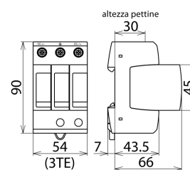
Dimensioni DG M YPV SCI 600
