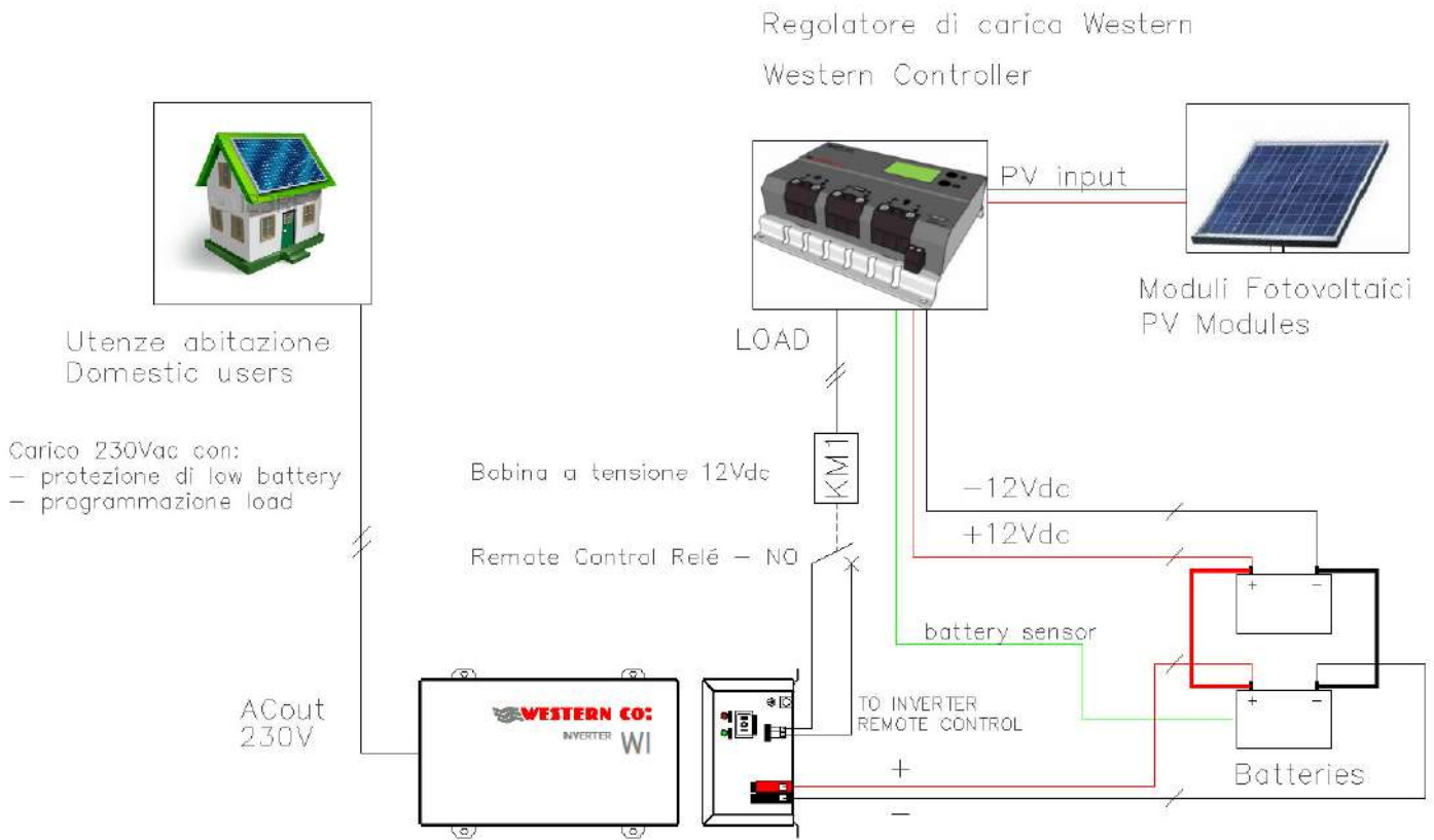
Fig. 3 Schema di collegamento WI400-12
