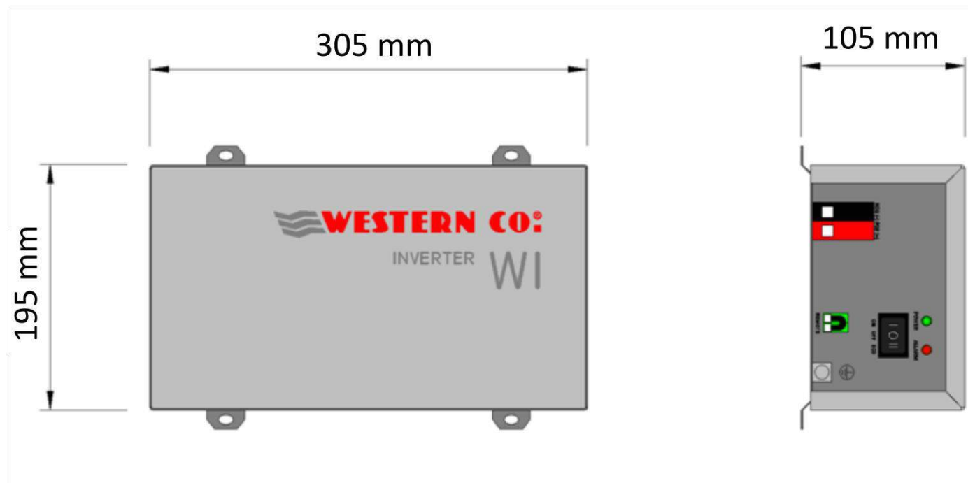
Fig. 5 Caratteristiche meccaniche
