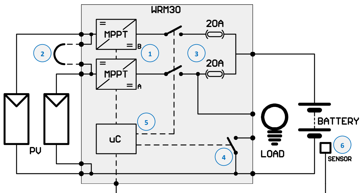
Fig. 1 Schema di principio
