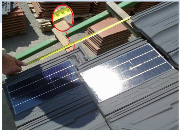
Passo tra tegola Ma.Xi.Ma. fotovoltaica e fotovoltaica circa 345 mm
